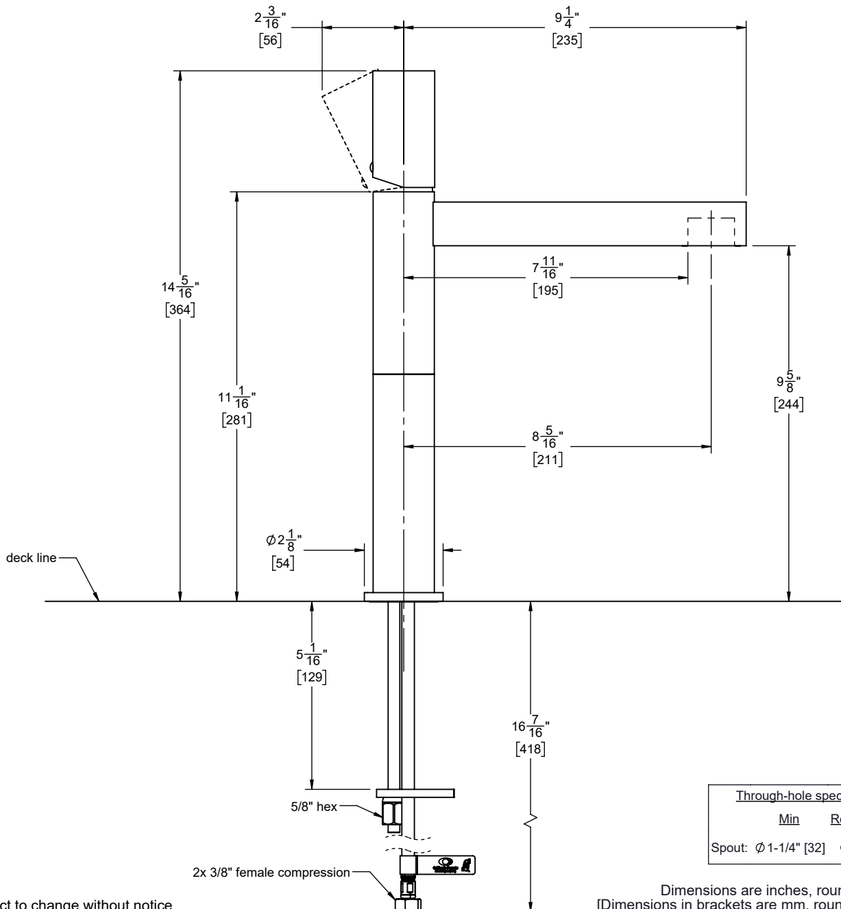
E301BCY-2 shown
