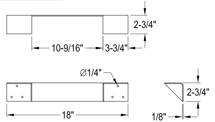
VSPLBRKT (1 pc)
